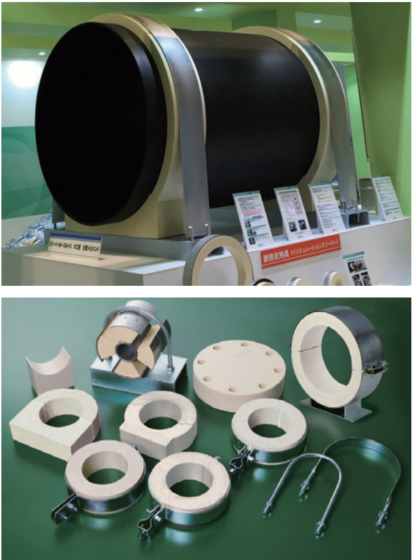
独自開発した断熱配管支持具「インシュレーションスリーパー」
